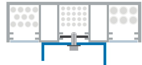
Das Profil als Halterung für zusätzliche Abhängungen o.Ä.
