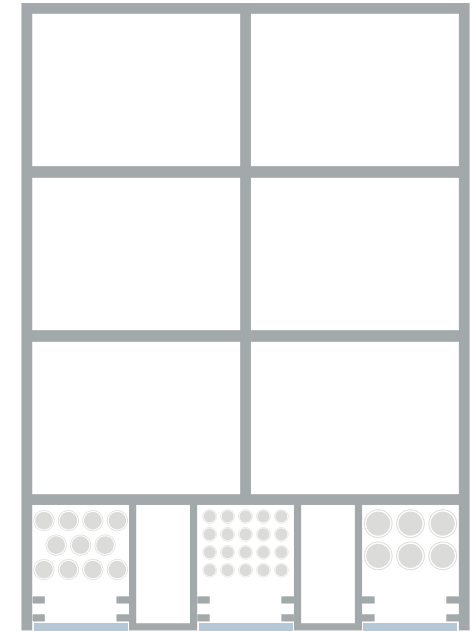
Unser Träger-Systemprofil (vereinfacht)
